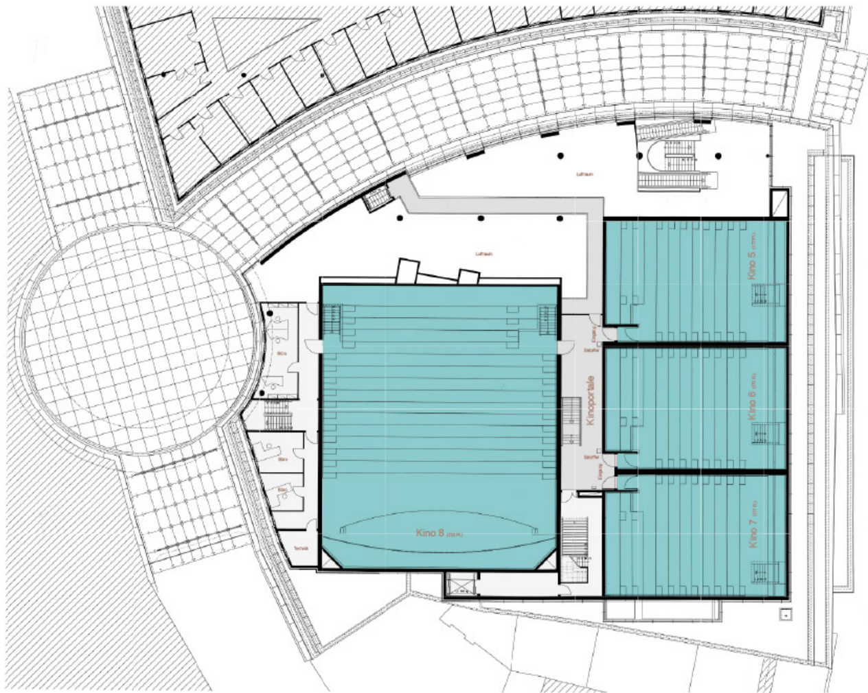
Grundriss: 5. OG
